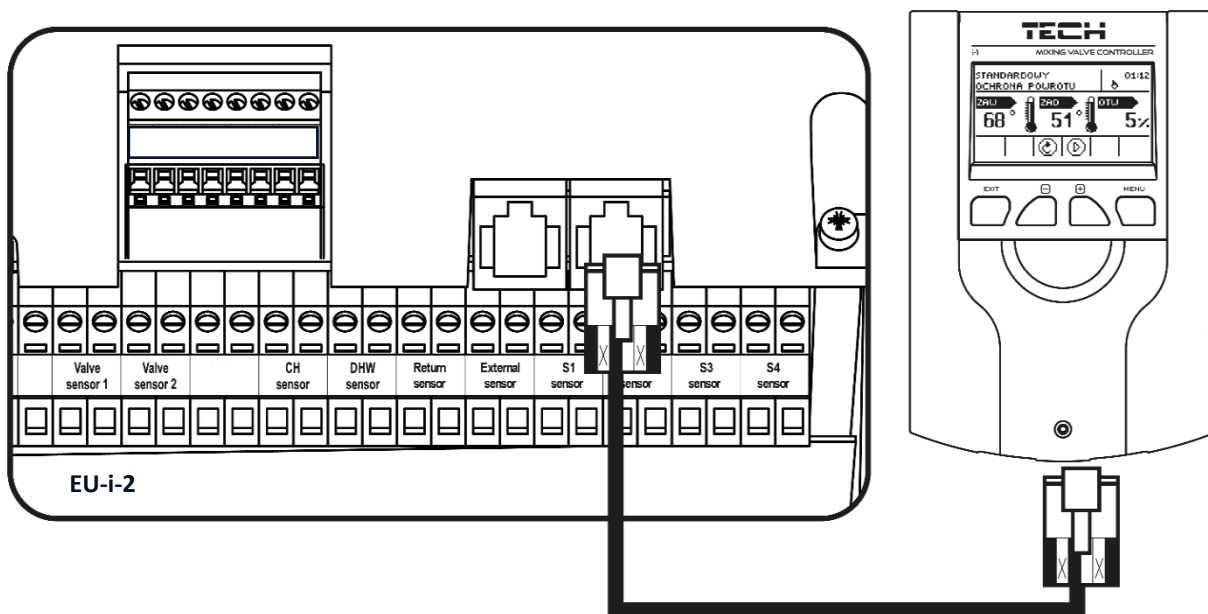
Példa: a pótszelep és az EU-i-2 fő vezérlő közötti kapcsolat
