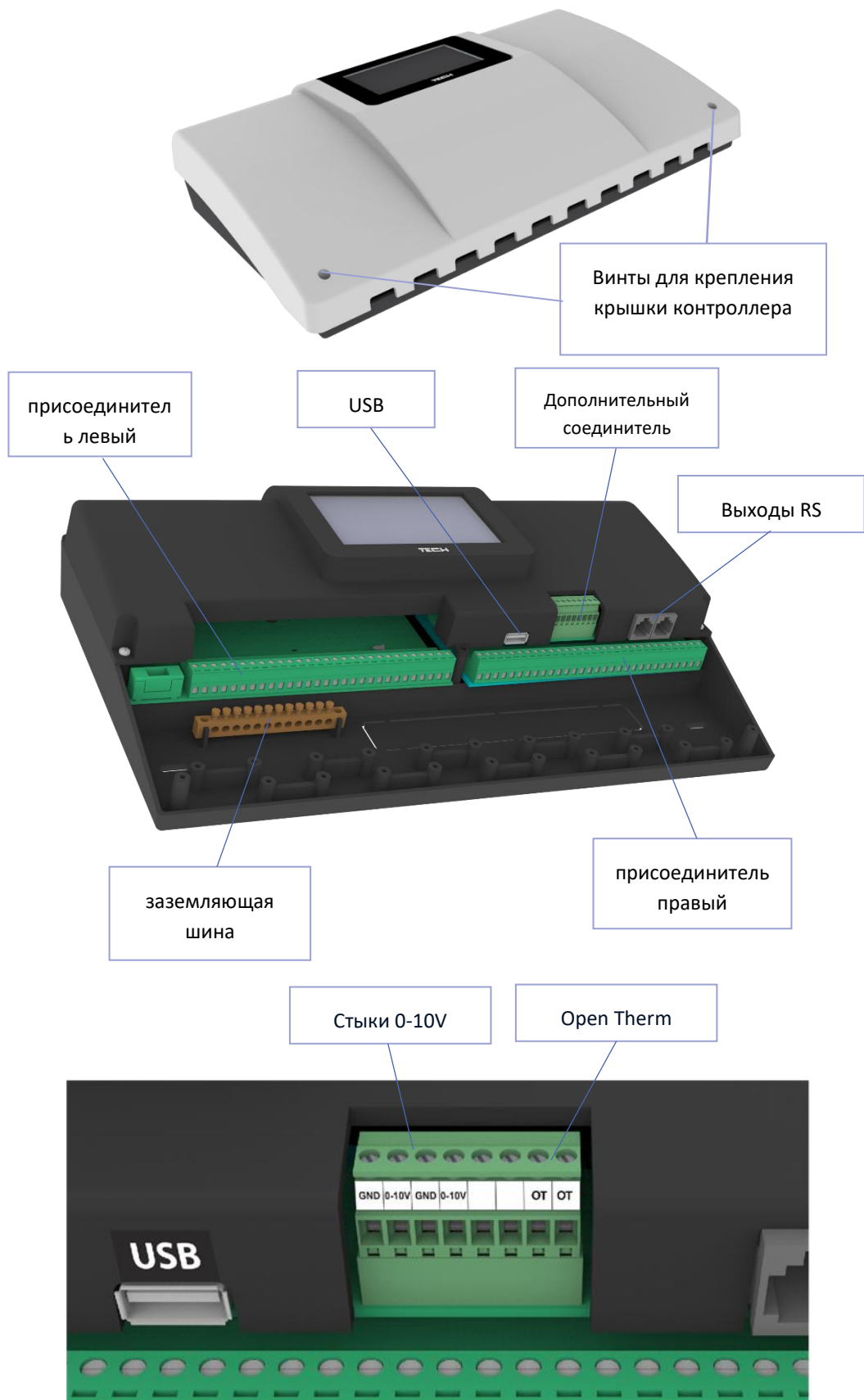
Соединитель стыков с напряжением 0 -10 V
