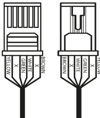
Примерное соединение дополнительного клапана с главным контроллером EU-I-2 Plus OT
