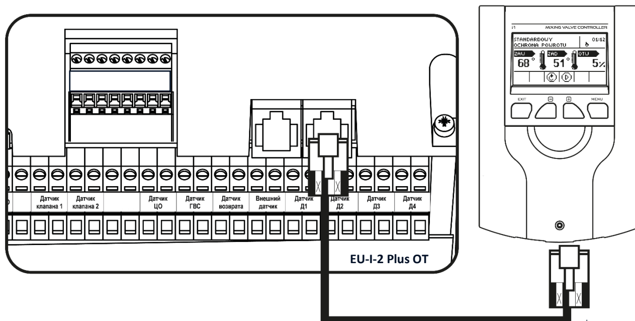
Примерное соединение дополнительного клапана с главным контроллером EU-I-2 Plus OT
