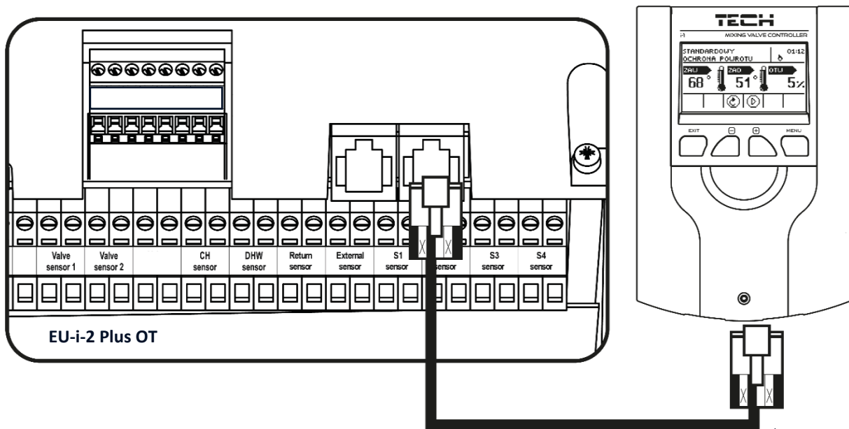
Példa: a pótszelep és az EU-i-2 Plus OT fő vezérlő közötti kapcsolat
