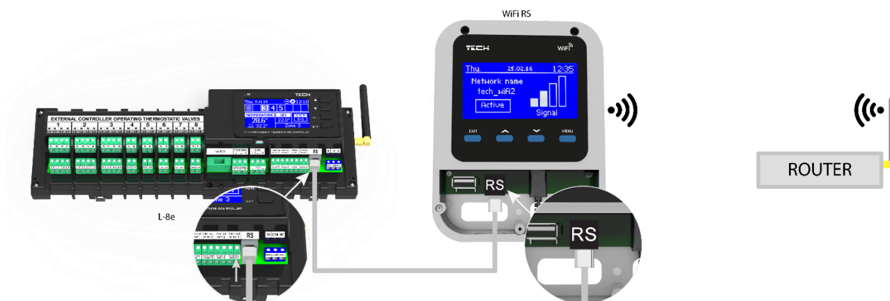
Kapcsolási rajz a WiFi RS-hez.
