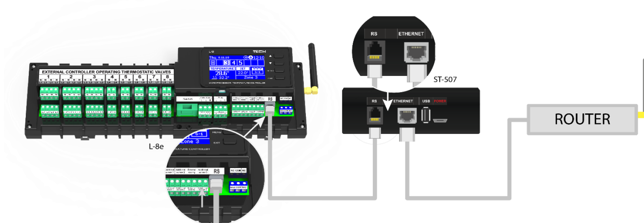
Kapcsolási rajz az ST-507 internetes modulhoz.
